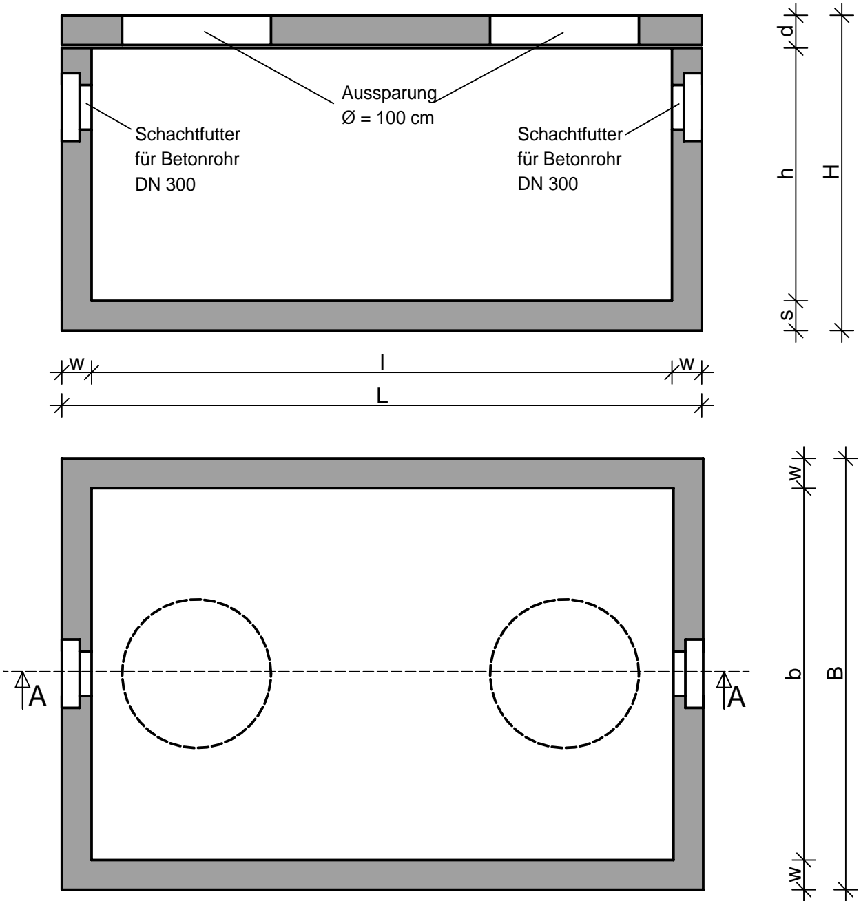
Schnitt A-A
