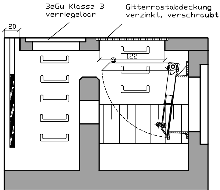
Schnitt A-A
