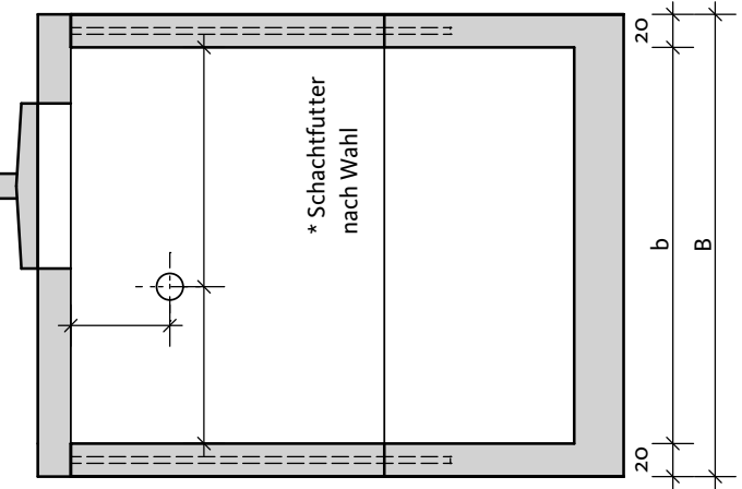
Schnitt C-C
