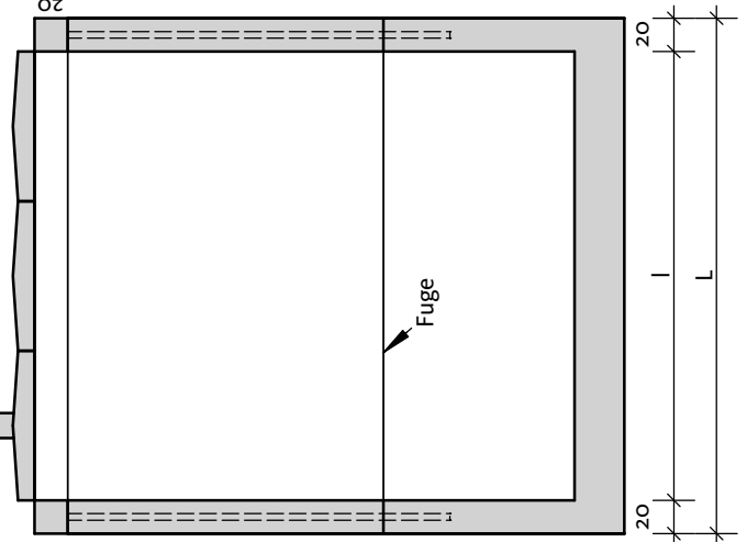
Schnitt A-A
