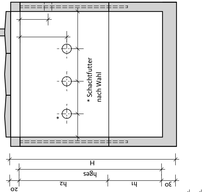
Schnitt B-B
